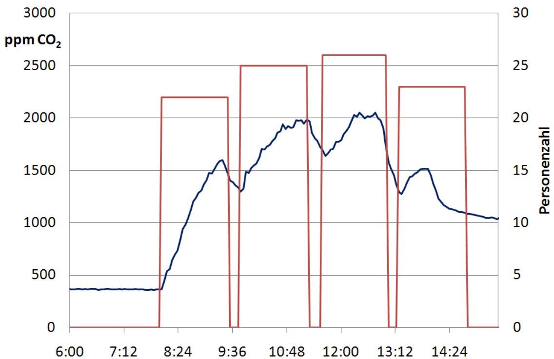
Abbildung 2-24: Konzentrationsverlauf TS38 bei geöffneten Oberlichtern
