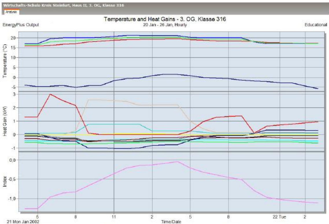
Abbildung 7-17: Verlauf der Wärmegewinne und -verluste, der Temperaturen und des Fanger-Index bei Nachtabsenkung im Ist-Zustand 34
