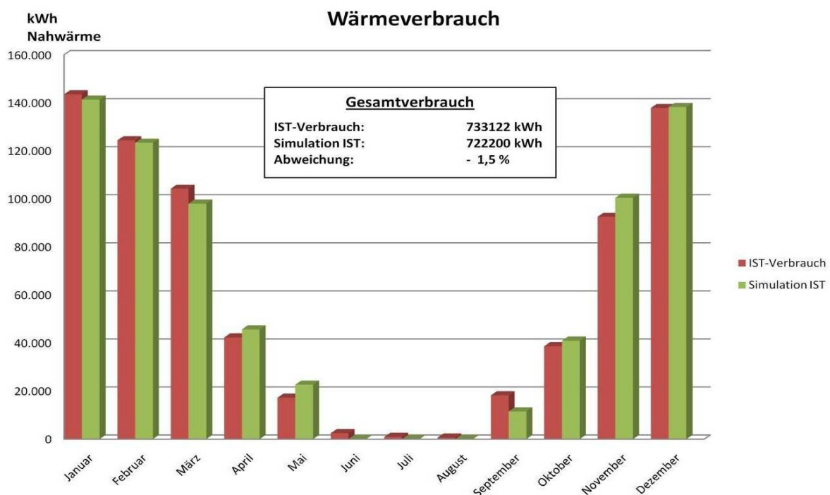
Abbildung 7-2: Vergleich vorhandener und simulierter Gesamtwärmeverbrauch der Technischen Schulen Steinfurt mit der Software DesignBuilder. Die Abweichung vom Ist-Wärmeverbrauch zur Simulation beträgt nur 1,5 %. 32
