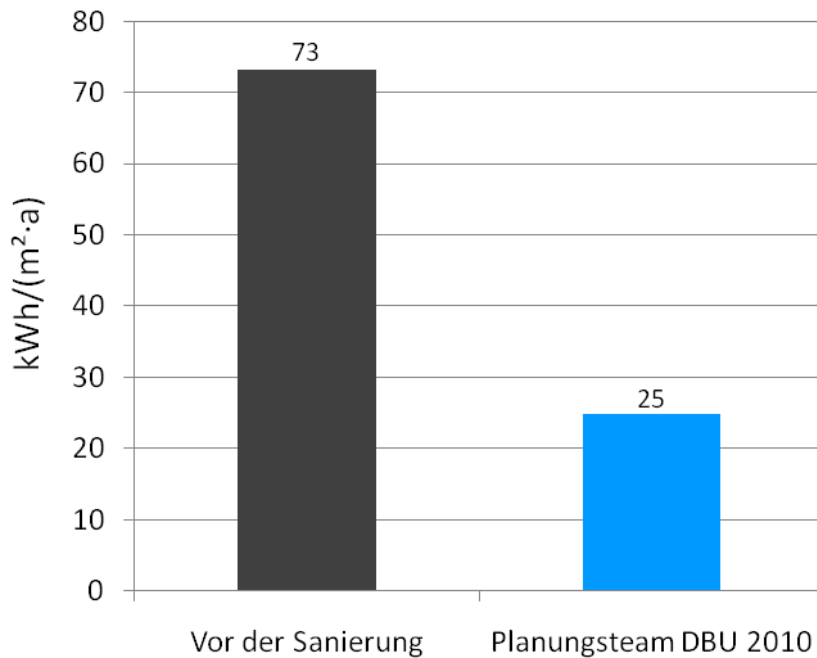
Abbildung 7-10: Vergleich des Jahresprimärenergieverbrauchs vor der Sanierung mit dem ermittelten Jahresprimärenergiebedarf nach Durchführung des Sanierungskonzept der Technischen Schulen, ermittelt mit DesignBuilder
