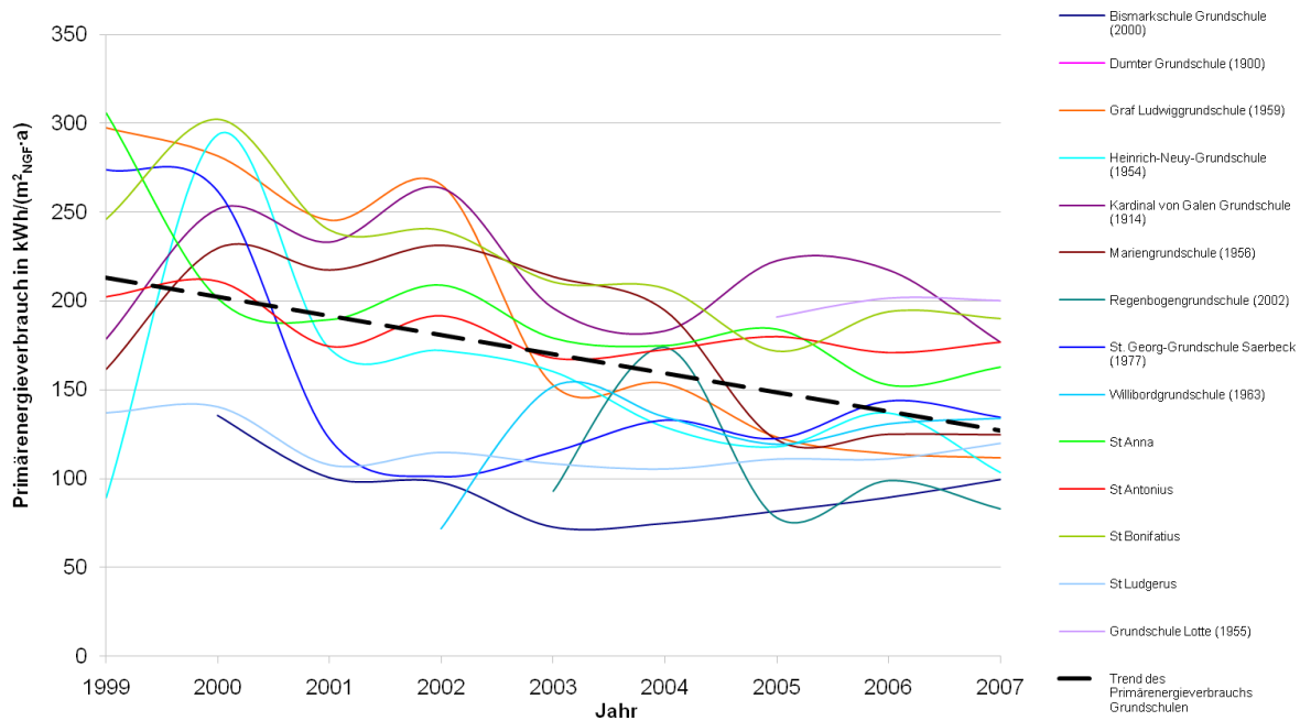
Abbildung 4-7: Primärenergieverbrauch in \text{kWh}/(\text{m}^2_{\text{NGF}}\cdot\text{a}) aller betrachteten Grundschulen (witterungsbereinigt, Standort: MS/OS)
