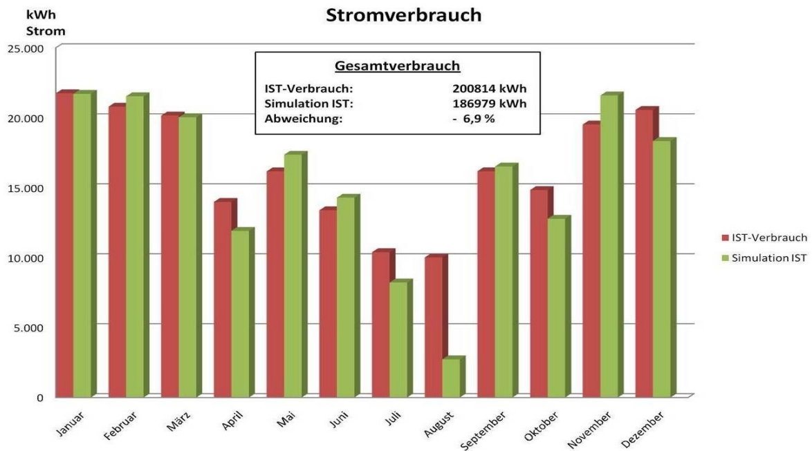
Abbildung 7-3: Vergleich vorhandener und simulierter Gesamtstromverbrauch der Technischen Schulen Steinfurt mit der Software DesignBuilder. Die Abweichung vom Ist-Stromverbrauch zur Simulation beträgt nur 6,9 %. 32
