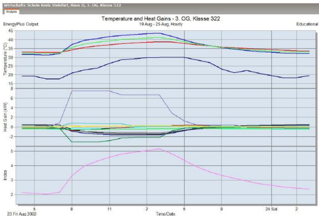
Abbildung 7-18: Verlauf der Temperaturen, Wärmegewinne und -verluste, Fanger-Index in einem ungekühlten Computerraum in Haus II 34
