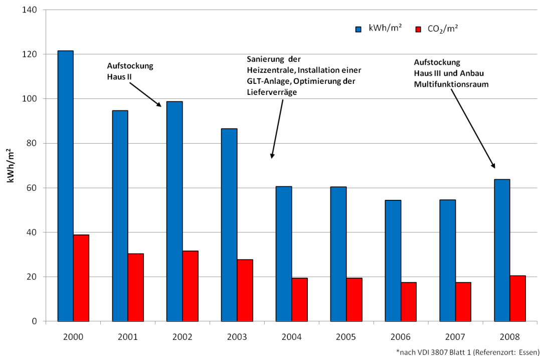
Abbildung 8-4: Witterungsbereinigter Verbrauch* pro m 2 der Wirtschaftsschulen Steinfurt mit der freigesetzten CO 2 Menge
