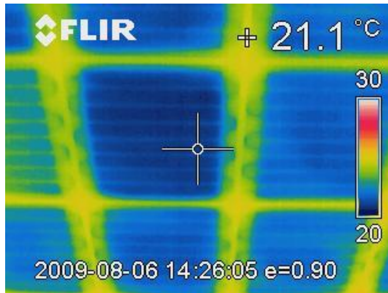
Abbildung 6-8: Thermografie-Aufnahme der Mäandern der Kühldecke
