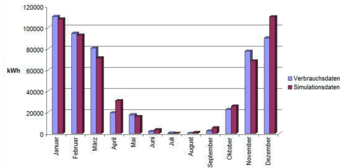
Abbildung 0-4: Vergleich des tatsächlichen Verbrauchs mit dem simulierten Verbrauch 1
