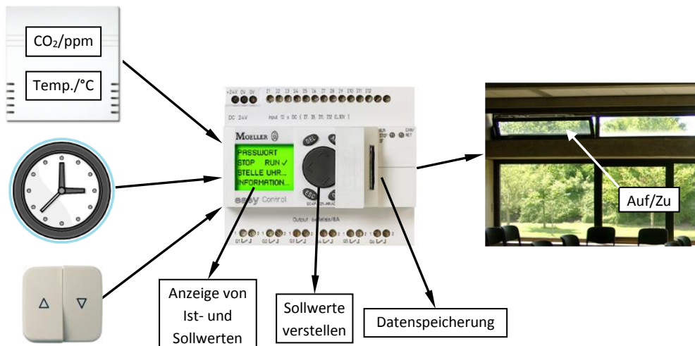
Abbildung 7-33: Funktionsweise der automatischen Fensterlüftung 37
