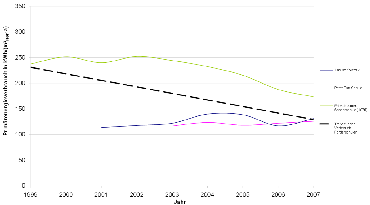
Abbildung 4-6: Primärenergieverbrauch in kWh/(m 2 NGF ·a) aller betrachteten Förderschulen (witterungsbereinigt, Standort: MS/OS)
