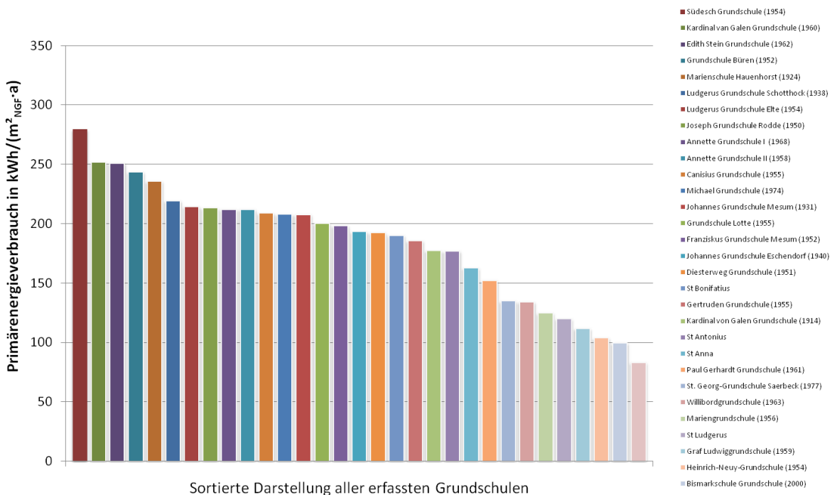
Abbildung 4-8: Sortierter Primärenergieverbrauch in \text{kWh}/(\text{m}^2_{\text{NGF}}\cdot\text{a}) aller erfassten Grundschulen für das Jahr 2007 (witterungsbereinigt)
