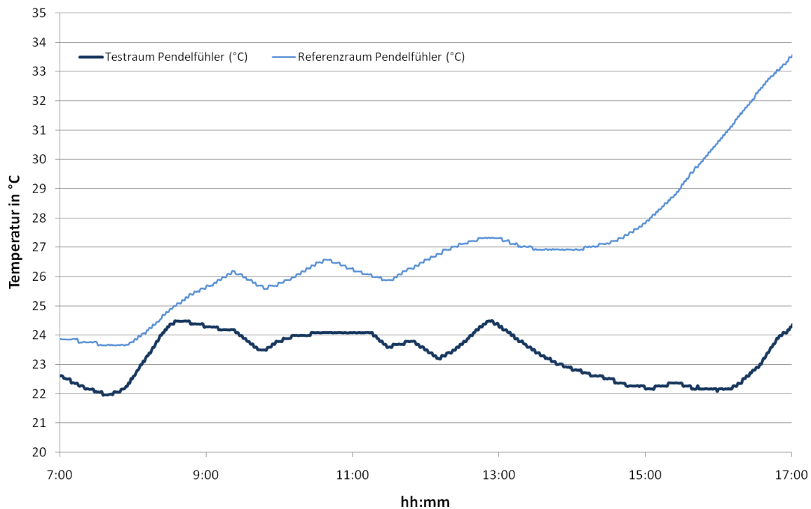
Abbildung 6-12: Raumlufttemperatur vom 24.08.09 beim Betrieb der Kühldecke in Raum 319 und im Referenzraum 326
