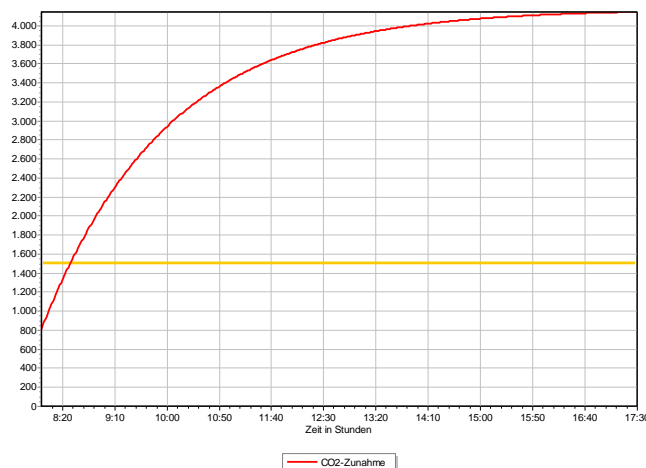
Abbildung 0-2: Verlauf der CO 2 -Konzentration berechnet mit der Software QUIRL/CO 2
