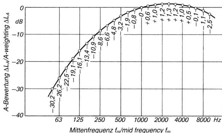
Abbildung 5-2: Korrekturwerte bei entsprechenden Mittenfrequenzen der Terzbänder nach VDI 2081
