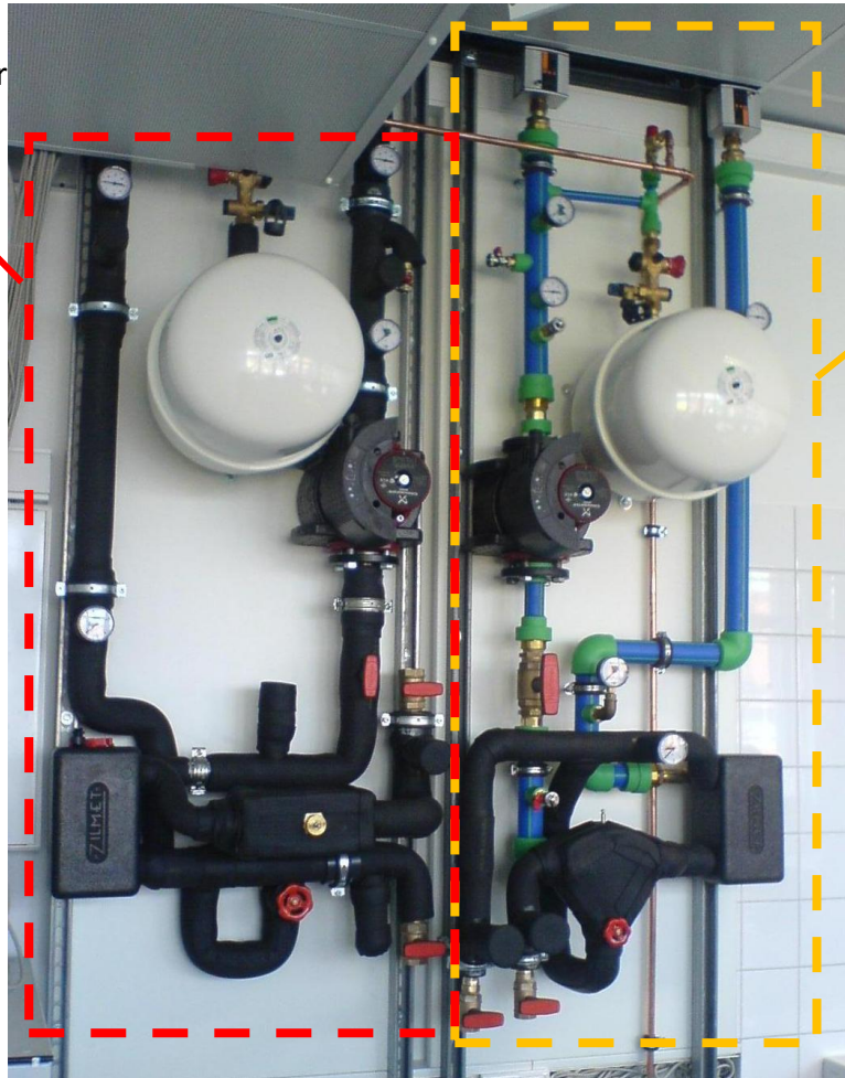
Abbildung 6-2: Übergabestation der Hochleistungskühldecke und der Schwerkraftkühlung in Raum 319 der Wirtschaftsschulen
