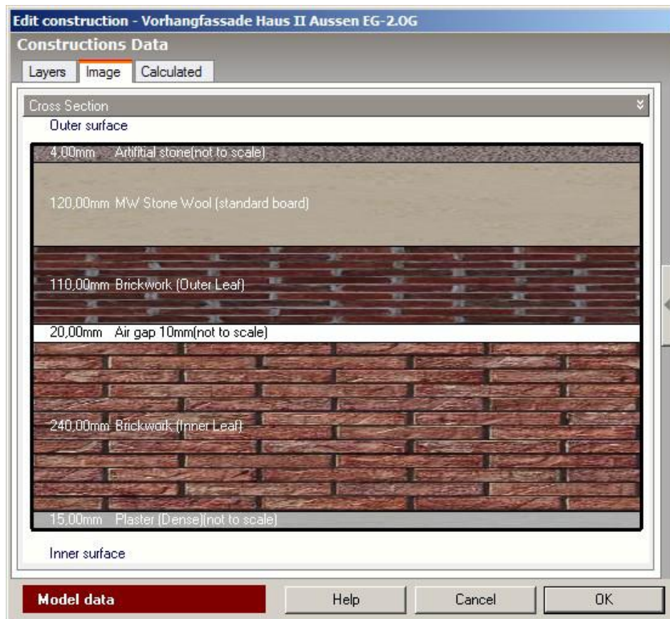
Abbildung 7-14: Aufbau der Außenwand mit Vorhangfassade 34
