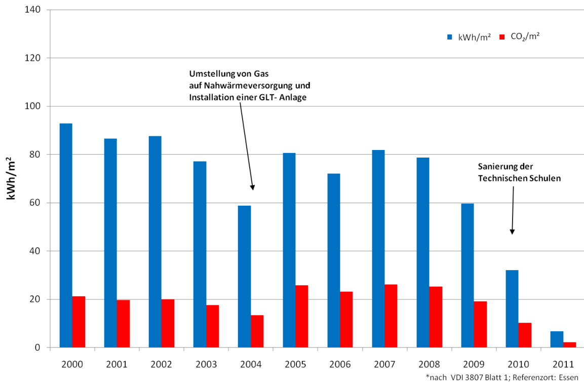
Abbildung 8-6: Witterungsbereinigter Verbrauch* pro m 2 der Technischen Schulen mit der freigesetzten CO 2 Menge bis zum Abschluss der Sanierung im Jahr 2011
