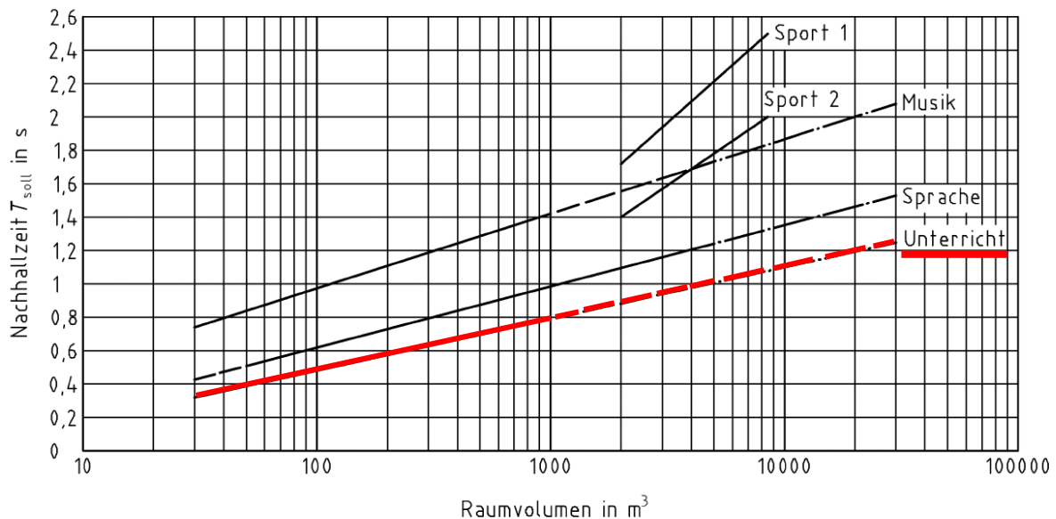
Abbildung 2-33: Sollwert T_{soll} der Nachhallzeit für unterschiedliche Nutzungsarten 9
