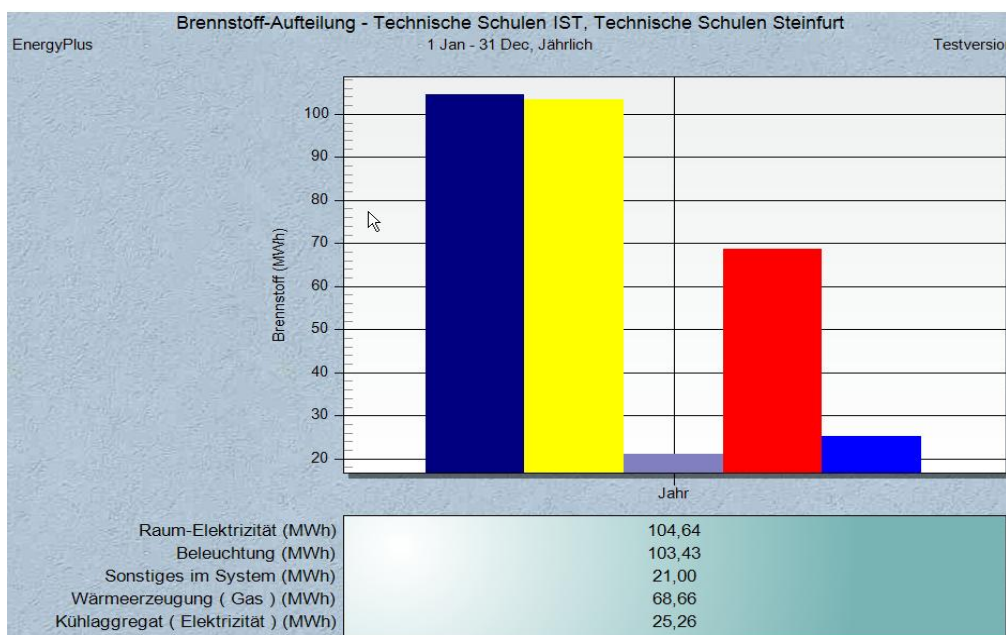
Abbildung 7-7: Detailliertes Berechnungsergebnis zur Brennstoff-Aufteilung der Technischen Schulen nach der Sanierung, dargestellt mit der Software DesignBuilder
