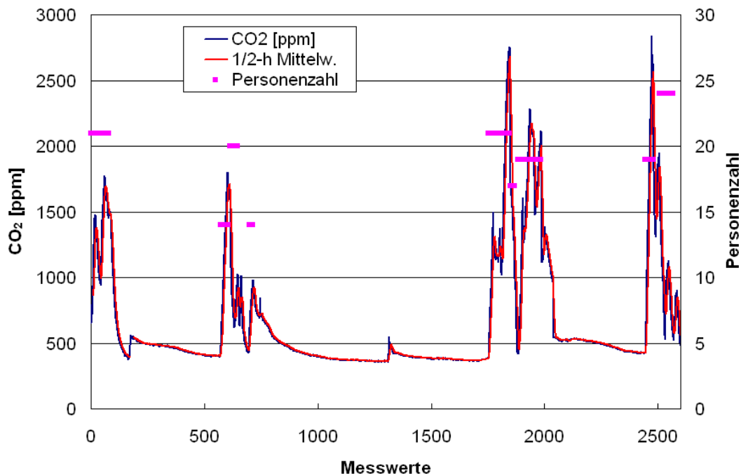
Abbildung 2-21: Vergleich von Einzelmessungen und gleitenden Halbstundenmittelwert der CO_2 -Konzentration in Raum WS111
