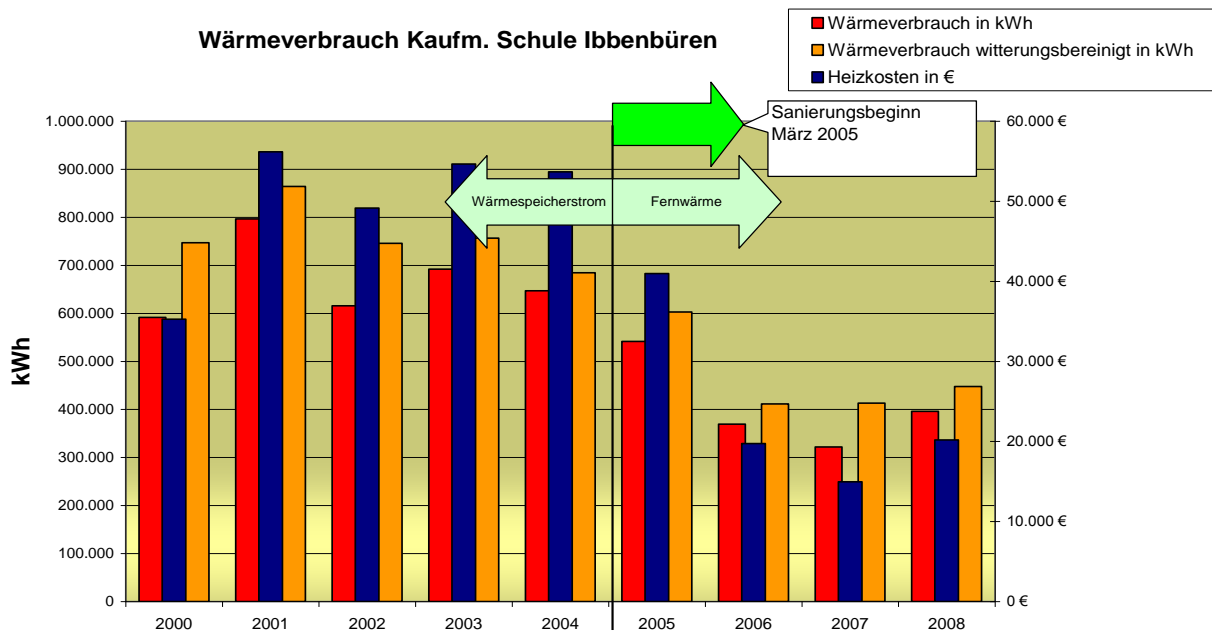
Abbildung 3-2: Betrachtung des Wärmeverbrauchs der Kaufmännischen Schulen Ibbenbüren, vor der Sanierung und nach der Sanierung mit Betreuung durch das Gebäudemanagement
