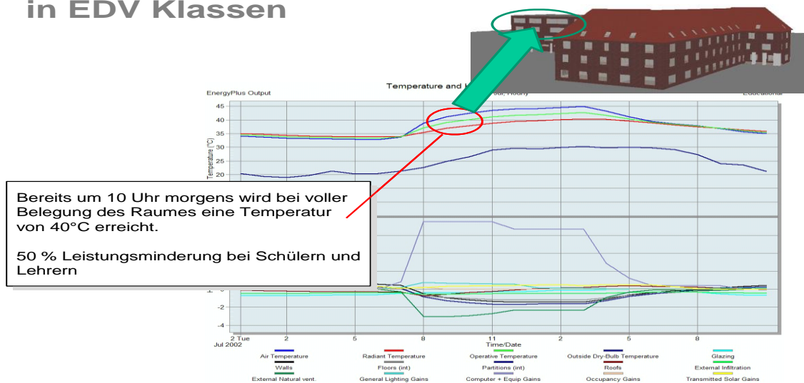
Abbildung 7-23: Ergebnisse einer dynamischen Simulation für einen EDV-Klassenraum einer Berufsschule 34
