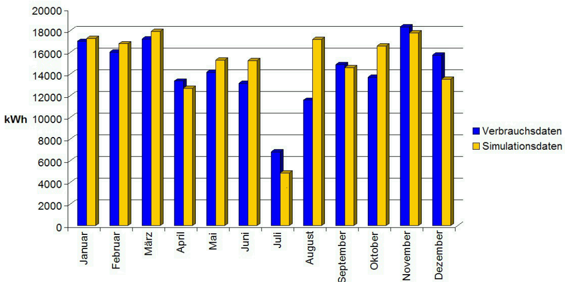
Abbildung 7-12: Monatlicher Stromverbrauch der Wirtschaftsschule – Vergleich von gemessenem und simuliertem Verbrauch 34
