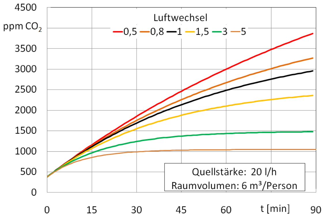
Abbildung 2-29: Einfluss des Luftwechsels auf die zeitliche Entwicklung der Kohlendioxidkonzentration
