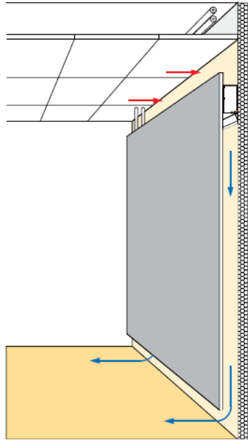
Abbildung 6-10: Schema des Funktionsprinzips der Schwerkraftkühlung
