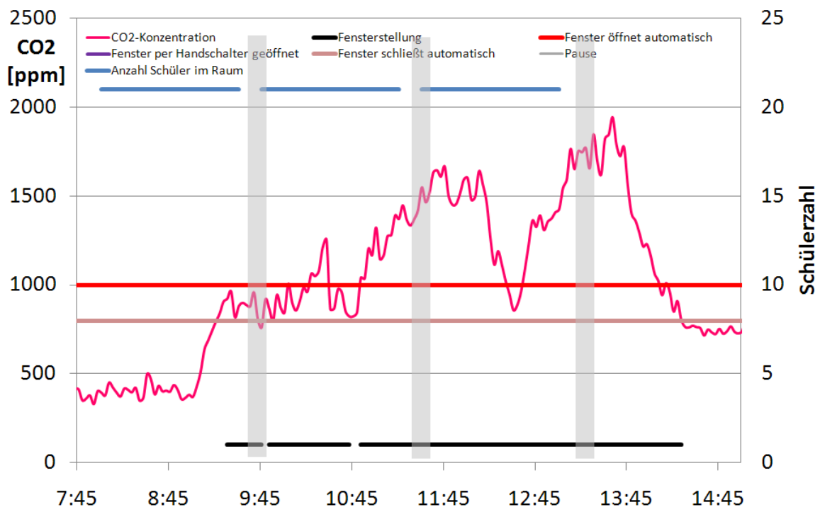
Abbildung 2-26: Auswirkungen eines automatischen Lüftungssystems
