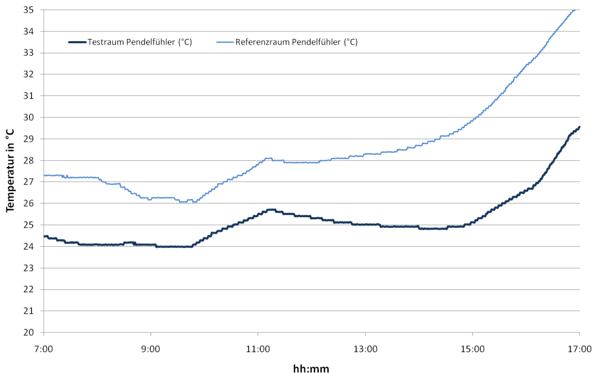
Abbildung 6-11: Raumlufttemperatur vom 19.08.09 beim Betrieb der Schwerkraftkühlung in Raum 319 und im Referenzraum 326
