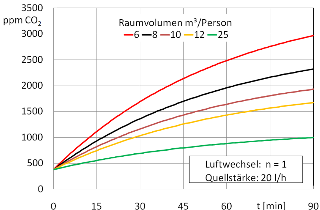
Abbildung 2-27: Einfluss des Raumvolumens auf die zeitliche Entwicklung der Kohlendioxidkonzentration
