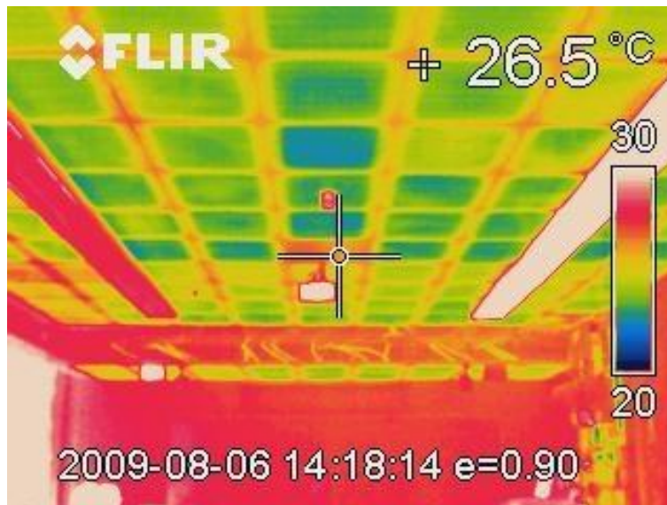
Abbildung 6-6: Thermografie-Aufnahme der Kühldecke in Raum 319 nach ca. 12 Minuten
