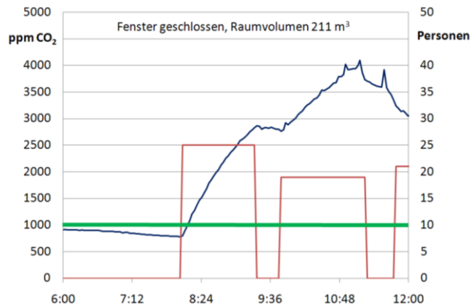
Abbildung 0-1: CO 2 -Konzentrationsverlauf in einem Klassenraum
