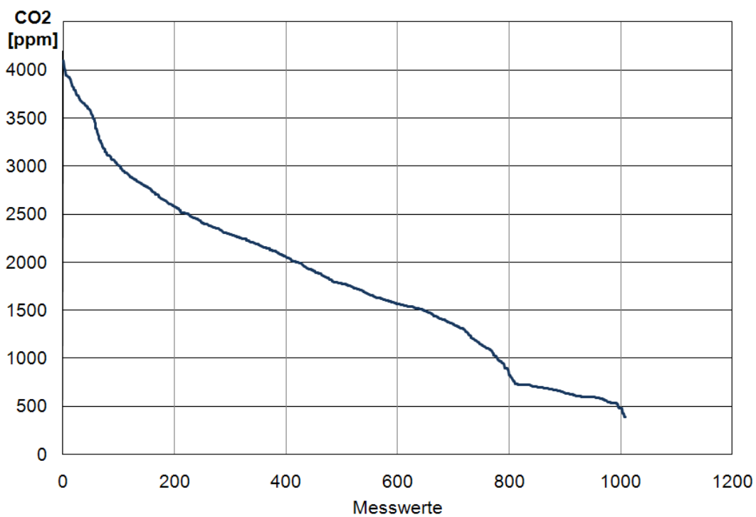
Abbildung 2-23: Nach Größe geordnete Konzentrationsmesswerte Raum TS136
