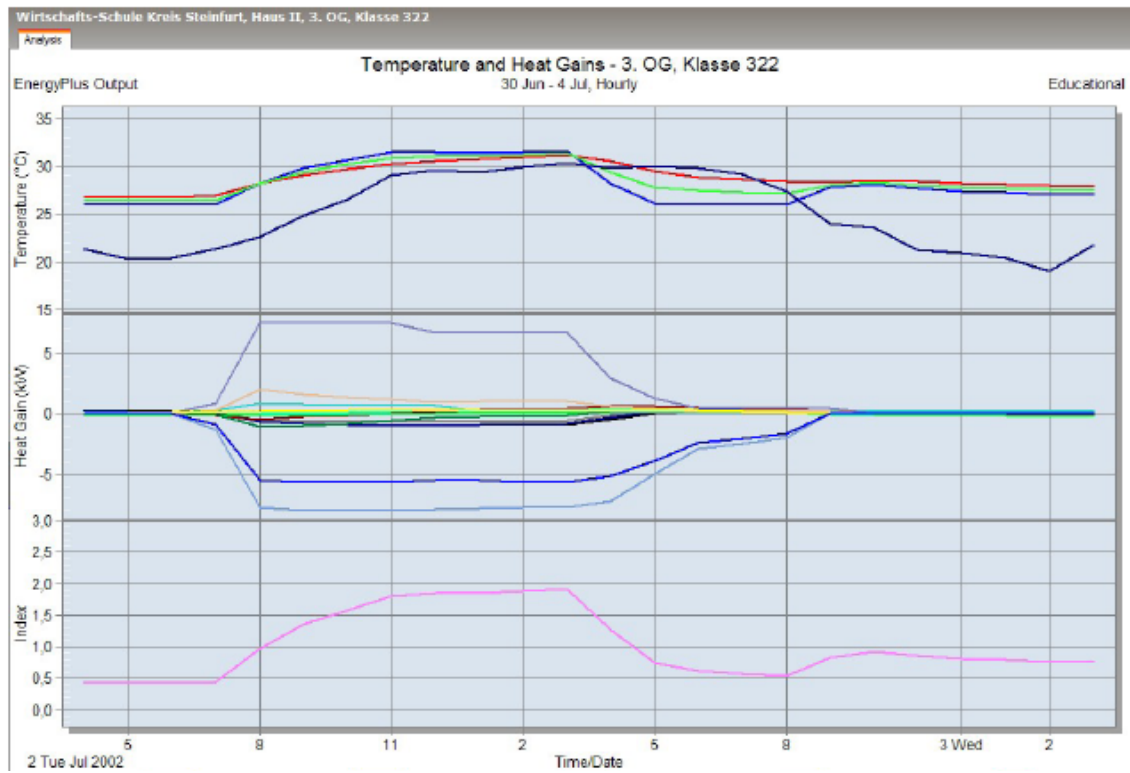
Abbildung 7-20: Verlauf der Temperaturen, Wärmegewinne und -verluste, Fanger-Index in einem gekühlten Computerraum in Haus II - Kühlleistung 6 kW 34
