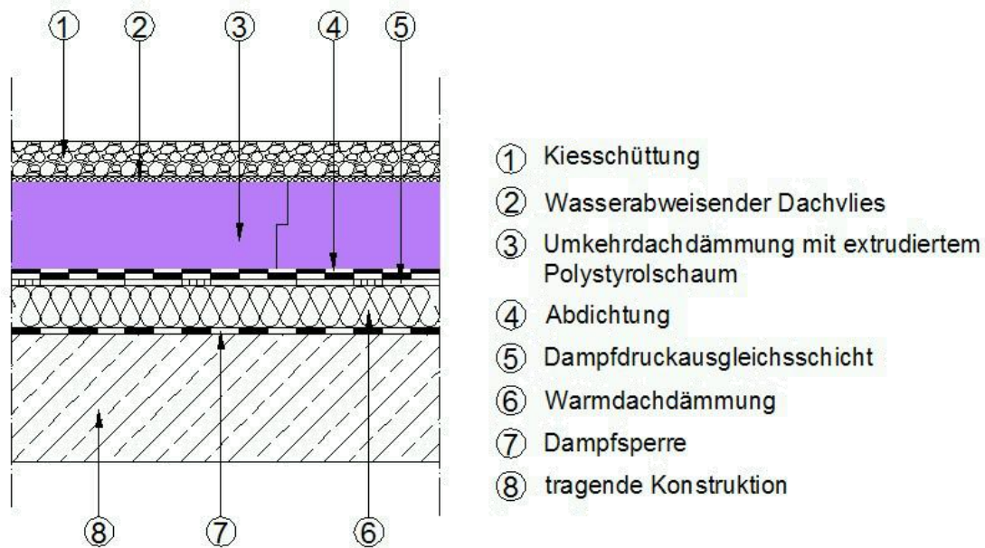
Abbildung 7-13: Dachaufbau der nachträglichen Dämmung am Haus I nach dem Umkehrdachsystem 35
