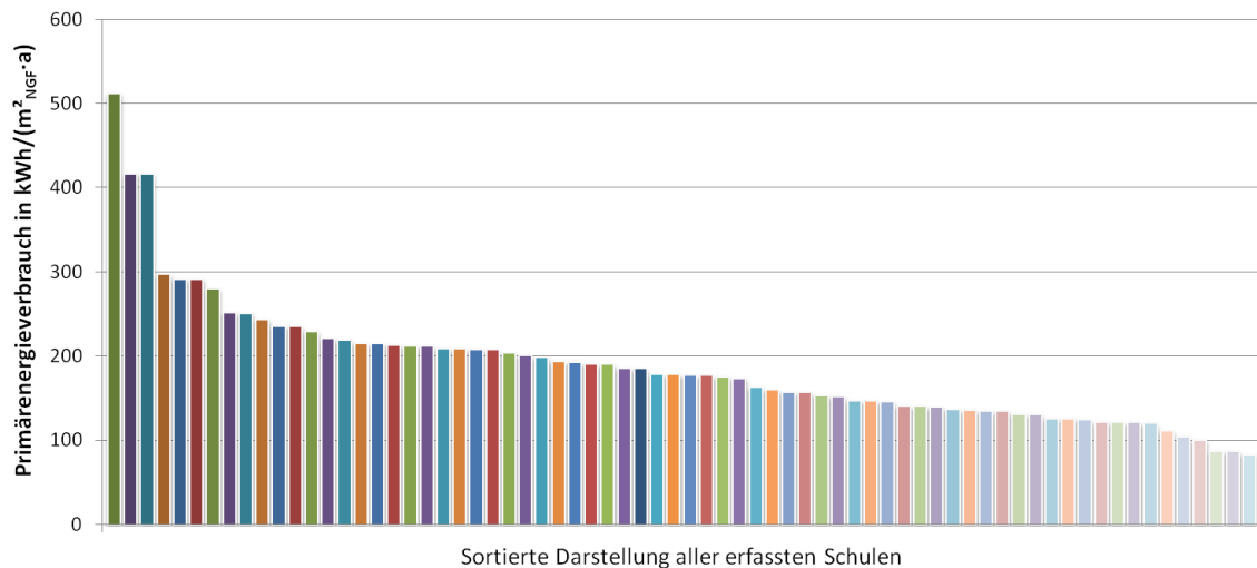
Abbildung 4-3: Sortierte Darstellung des Primärenergieverbrauchs in kWh/(m 2 NGF ·a) aller erfassten Schulen für das Jahr 2007 (witterungsbereinigt)
