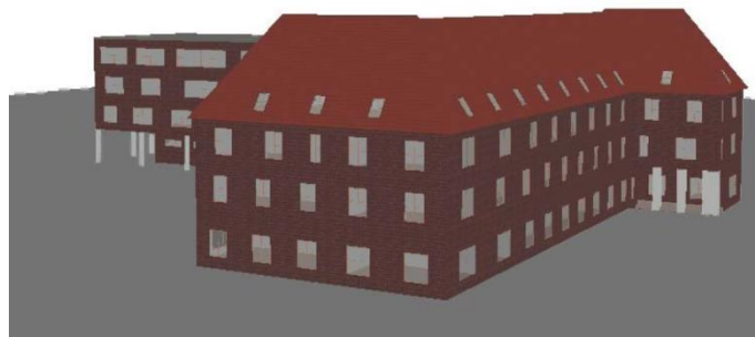
Abbildung 0-3: Darstellung der Wirtschaftsschulen mit der Software DesignBuilder für die thermische Gebäudesimulation 1
