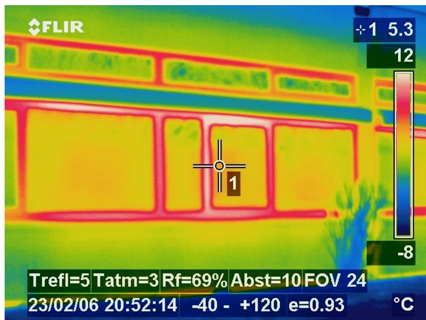
Abbildung 2-18: Technische Schulen Steinfurt – Thermografie Ansicht Nordfassade zeigt bereits isolierverglaste Fensterscheiben. Die Fensterprofile und besonders die Betonbalken sind hingegen ohne jegliche Dämmung.
