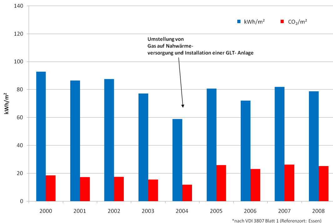
Abbildung 8-5: Witterungsbereinigter Verbrauch* pro m 2 der Technischen Schulen Steinfurt mit der freigesetzten CO 2 Menge
