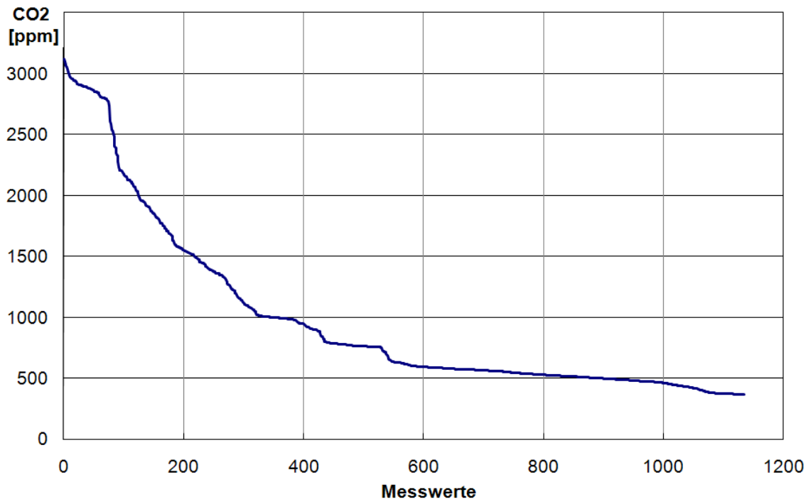
Abbildung 2-22: Nach Größe geordnete Konzentrationsmesswerte Raum TS17
