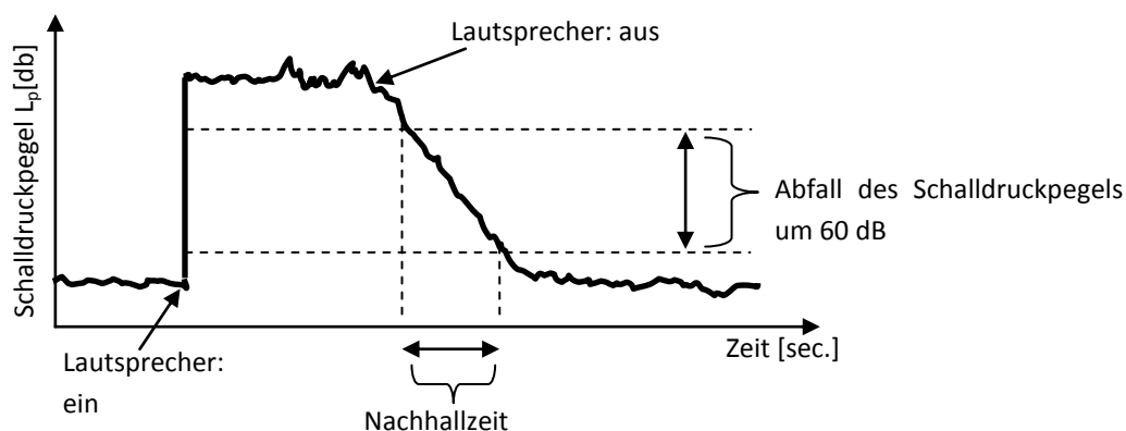
Abbildung 5-3: Messverlauf zur Ermittlung der Nachhallzeit
