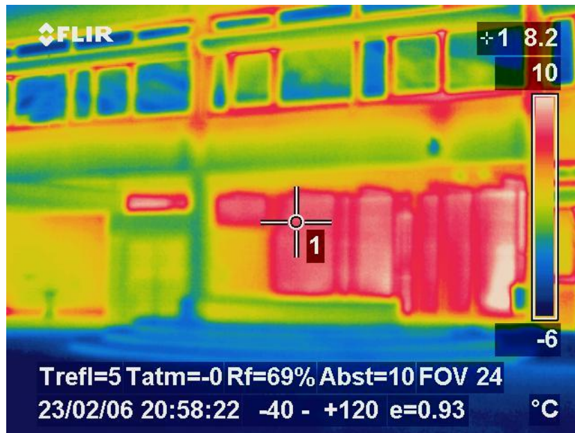
Abbildung 2-17: Technische Schulen Steinfurt – Thermografie der Ansicht des Haupteingangsbereich mit Einscheibenverglasung. Es zeigt sich die bauphysikalische Mängelsituation im Bereich der ungedämmten Fensterprofile und der fehlenden Dämmungen im Bereich der Stützen und Balken.
