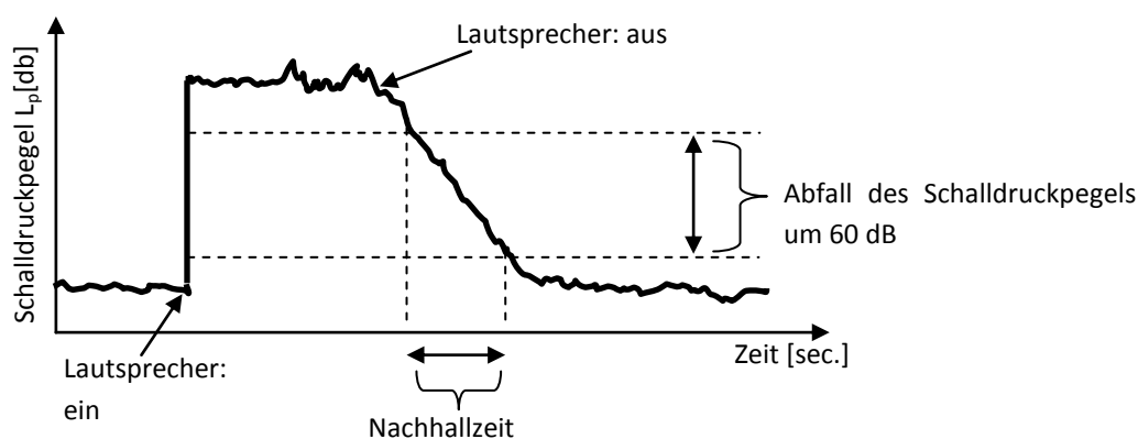
Abbildung 2-32: Messverlauf zur Ermittlung der Nachhallzeit
