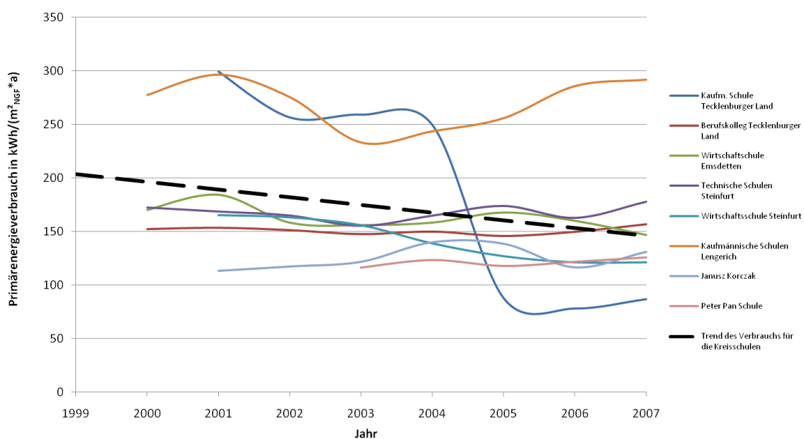
Abbildung 3-1: Primärenergieverbrauch in kWh/(m 2 NGF ·a) der Kreisschulen (witterungsbereinigt, Standort: MS/OS)
