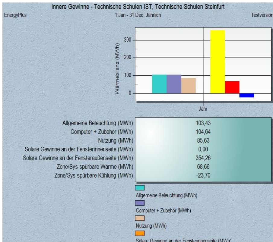
Abbildung 7-8: Detailliertes Berechnungsergebnis der inneren Gewinne der Technischen Schulen nach der Sanierung, dargestellt mit der Software DesignBuilder
