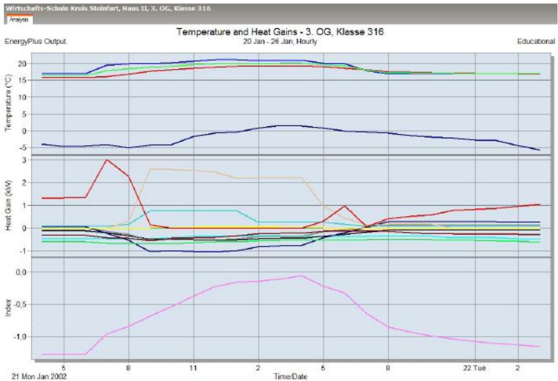
Abbildung 7-16: Verlauf der Wärmegewinne und -verluste, der Temperaturen und des Fanger-Index bei verlängerter Nachtabsenkung 34
