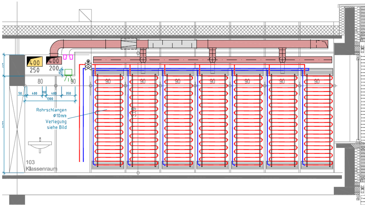
Abbildung 7-26: Detailzeichnung der Klimawand
