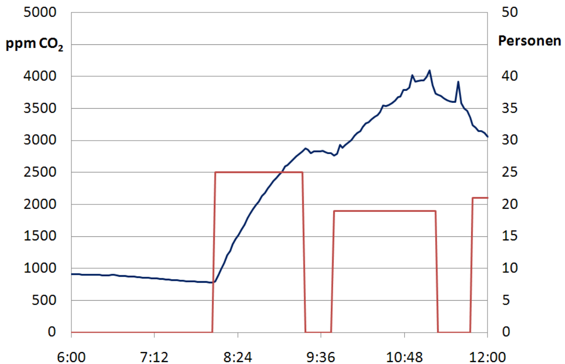
Abbildung 2-25: Konzentrationsverlauf TS136 bei geschlossenen Fenstern
