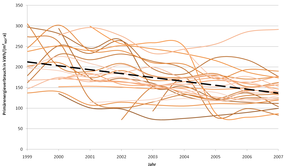
Abbildung 4-2: Primärenergieverbrauch in kWh/(m 2 NGF ·a) für alle betrachteten Schulen (witterungsbereinigt, Standort: MS/OS)
