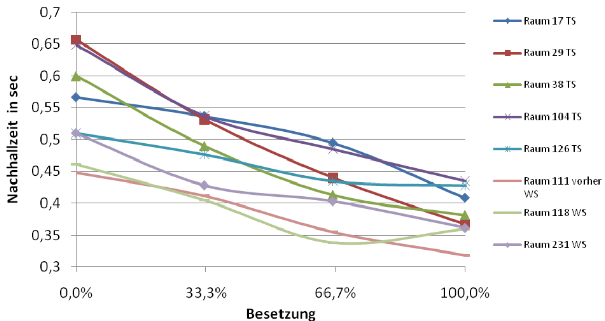
Abbildung 2-49: Nachhallzeit in Abhängigkeit der Besetzung für alle untersuchten Klassenräume
