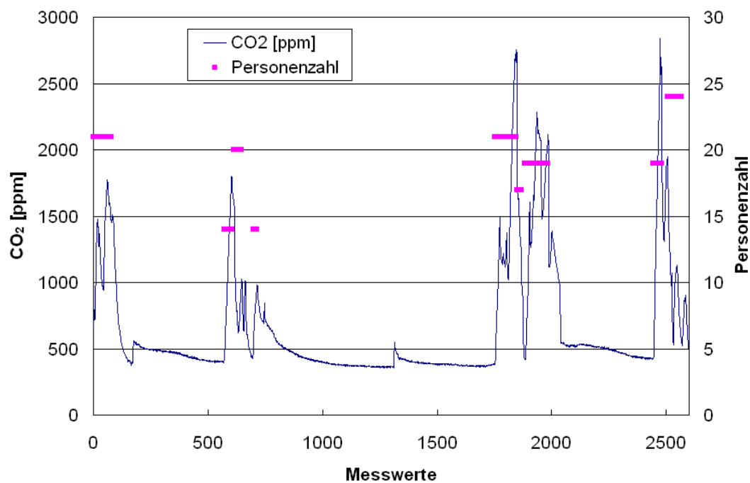
Abbildung 2-20: Im Messzeitraum gemessene CO 2 -Konzentration in Raum WS111
