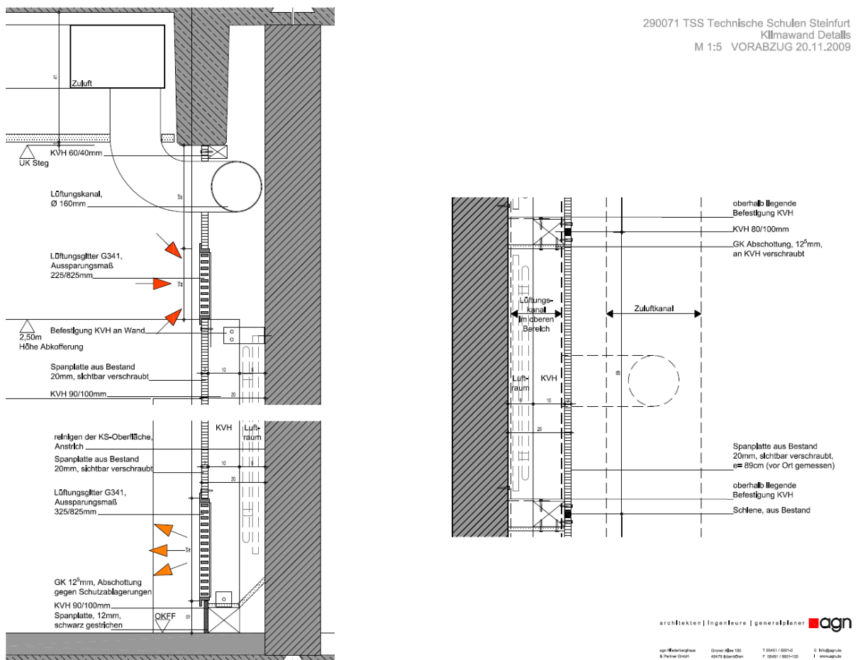
Abbildung 7-27: Technische Detailzeichnungen der Klimawand
