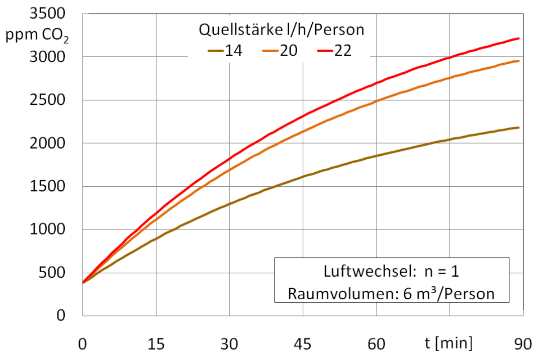
Abbildung 2-28: Einfluss der Quellstärke auf die zeitliche Entwicklung der Kohlendioxidkonzentration
