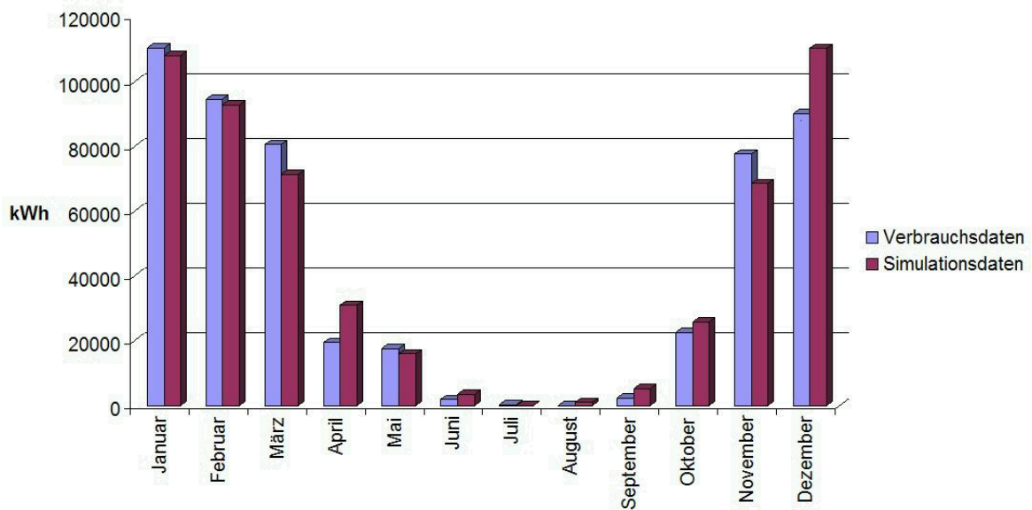
Abbildung 7-11: Monatlicher Nutzwärmeverbrauch der Wirtschaftsschule – Vergleich von gemessenem und simuliertem Verbrauch 34
