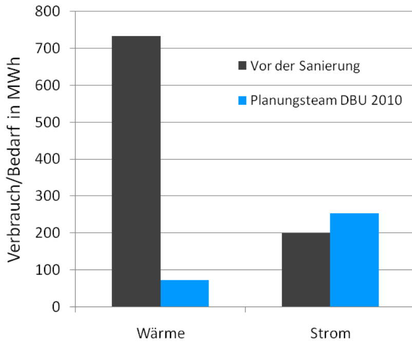
Abbildung 7-9: Vergleich des Wärme- und Stromverbrauchs vor der Sanierung mit dem simulierten Bedarf nach Durchführung der geplanten Sanierungsmaßnahmen für die Technischen Schulen, ermittelt mit DesignBuilder
