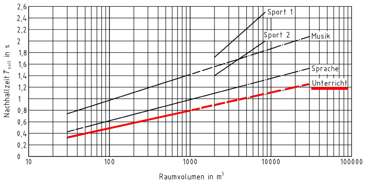
Abbildung 5-4: Sollwert T_{soll} der Nachhallzeit für unterschiedliche Nutzungsarten 31
