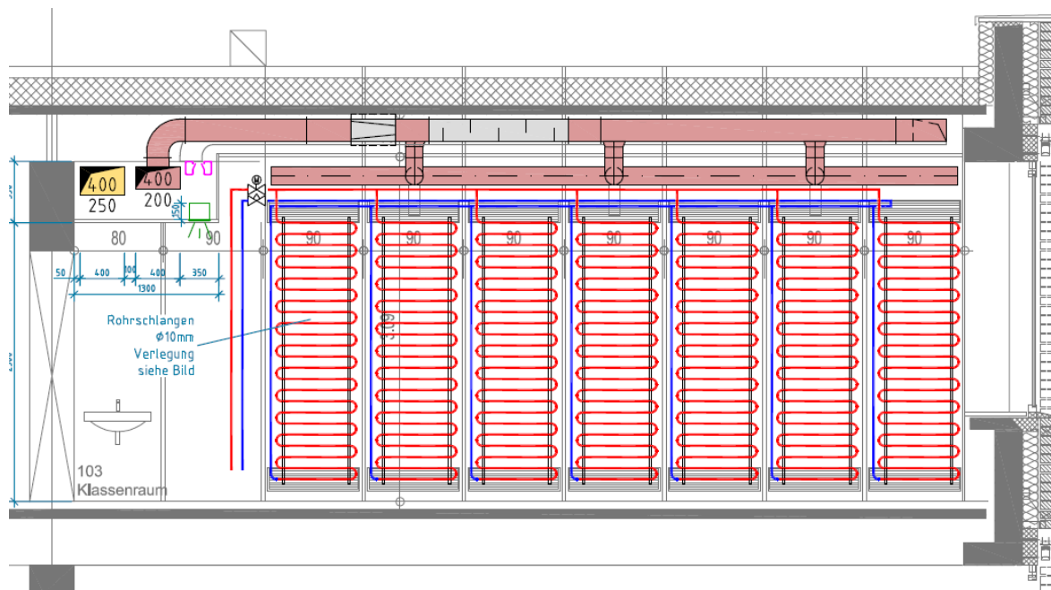
Abbildung 8-1: Detailzeichnung der Klimawand
