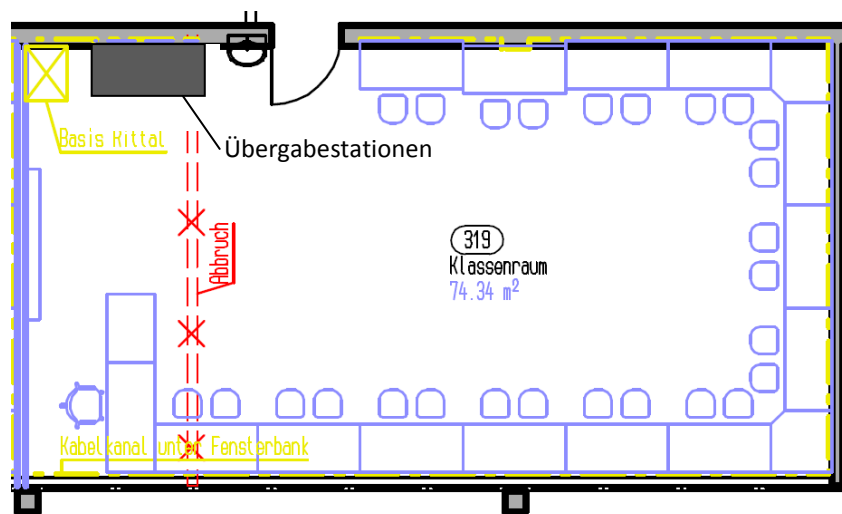
Abbildung 6-1: Position der Übergabestation der Hochleistungsdecke und der Schwerkraftkühlung in Raum 319 der Wirtschaftsschulen
