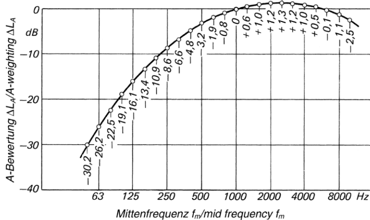
Abbildung 2-31: Korrekturwerte bei entsprechenden Mittenfrequenzen der Terzbänder nach VDI 2081
