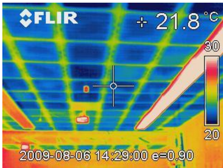
Abbildung 6-7: Thermografie der Kühldecke in Raum 319 nach ca. 25 Minuten
