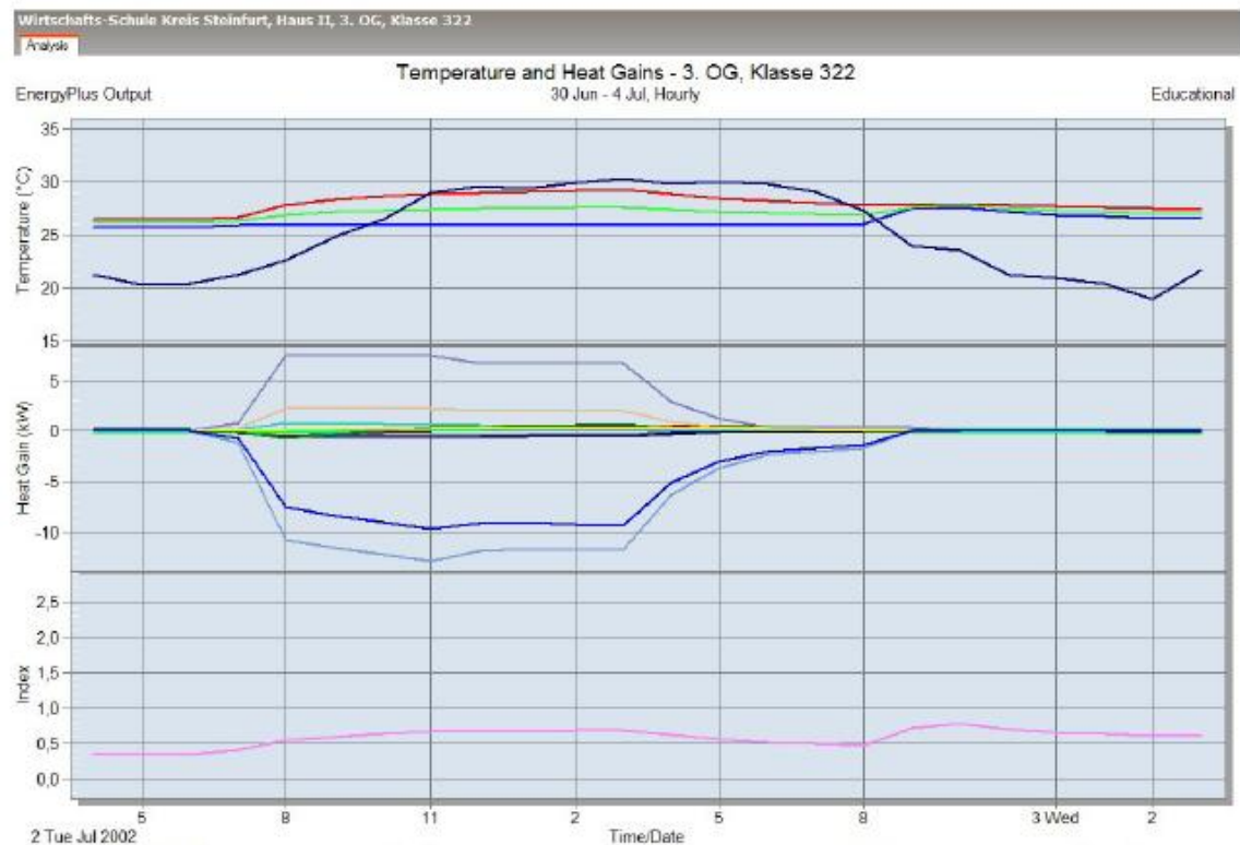
Abbildung 7-19: Verlauf der Temperaturen, Wärmegewinne und -verluste, Fanger-Index in einem gekühlten Computerraum in Haus II - Kühlleistung 10 kW 34
