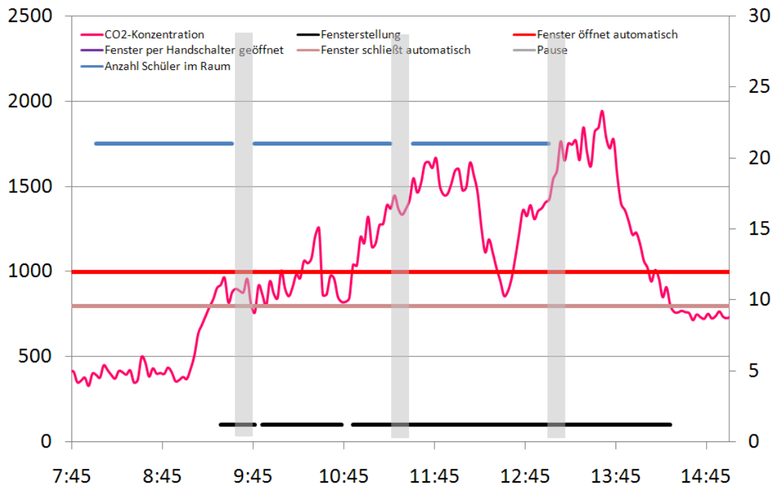
Abbildung 7-35: Auswirkungen eines automatischen Lüftungssystem
