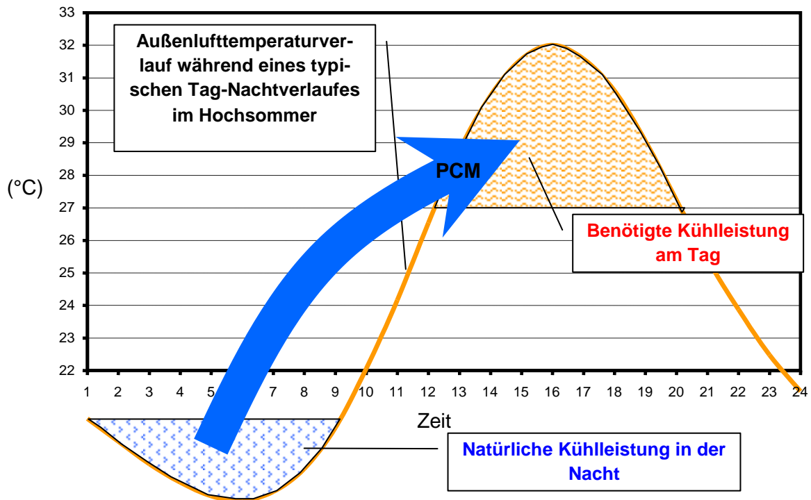
Abbildung 7-31: Grafische Darstellung des sommerlichen Kühlfalls während eines typischen Tag-Nachtverlaufes. Die Wärme, die nachts vom PCM abgegeben wird, kann tagsüber zur Kühlung der Zuluft in einem zentralen oder dezentralen Energiespeicher wieder aufgenommen werden.
