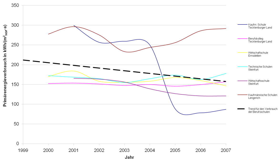
Abbildung 4-4: Primärenergieverbrauch in kWh/(m 2 NGF ·a) aller betrachteten Berufsschulen (witterungsbereinigt, Standort: MS/OS)
