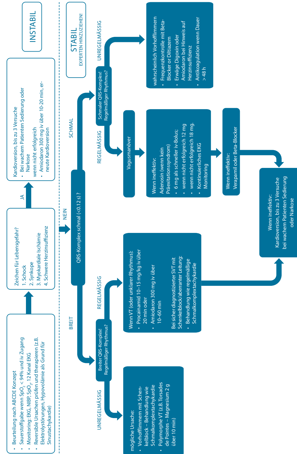
Abbildung 11 Tachykardie-Algorithmus
